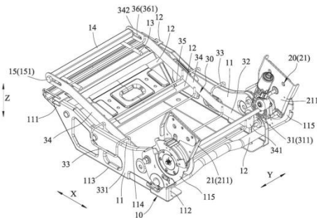
座椅結構圖示
